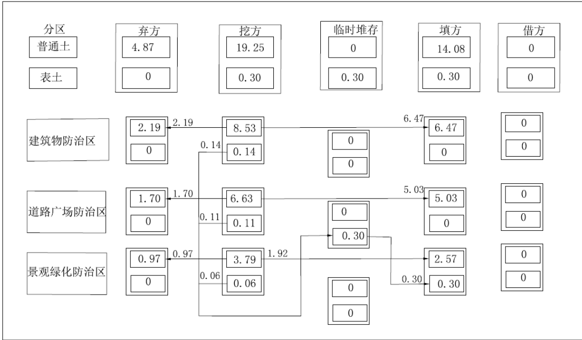
图 3-1 工程土石方流向
